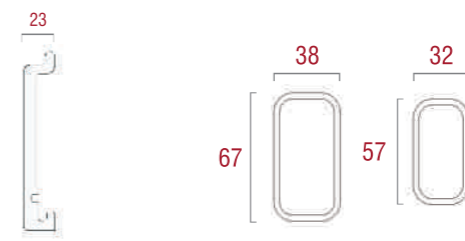
profilo bracci "tipo B" "B" type arms profile
